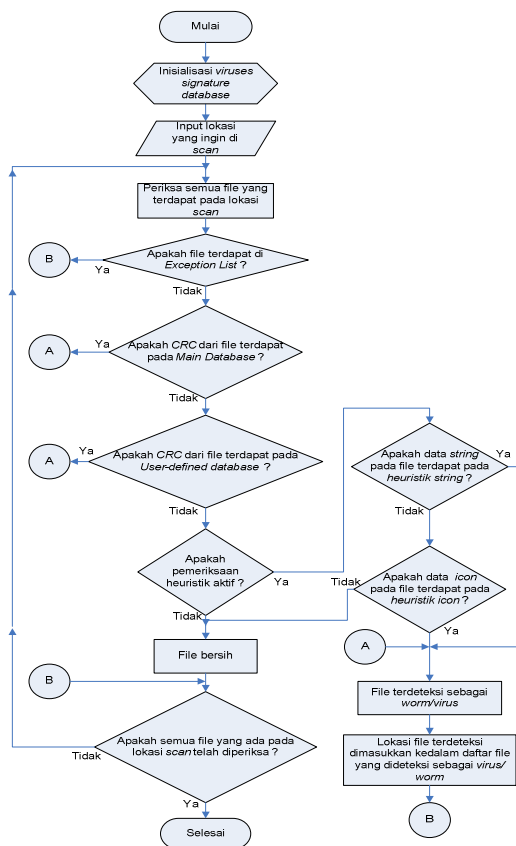
Gambar 17. Flowchart proses scanning pada software antivirus yang dibuat
