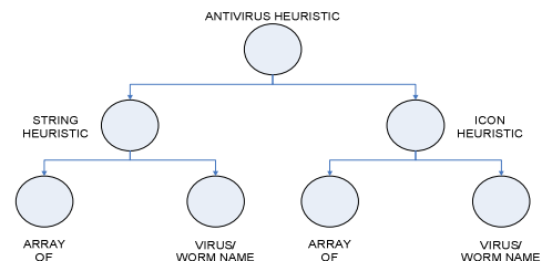
Gambar 16. Pohon heuristik yang digunakan pada software antivirus ini
